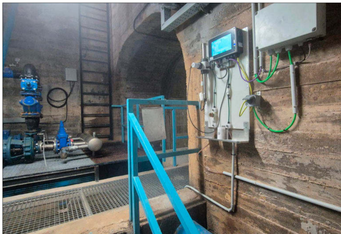
Instalación de sensorización realizada por Aguas de Burgos. ECB
